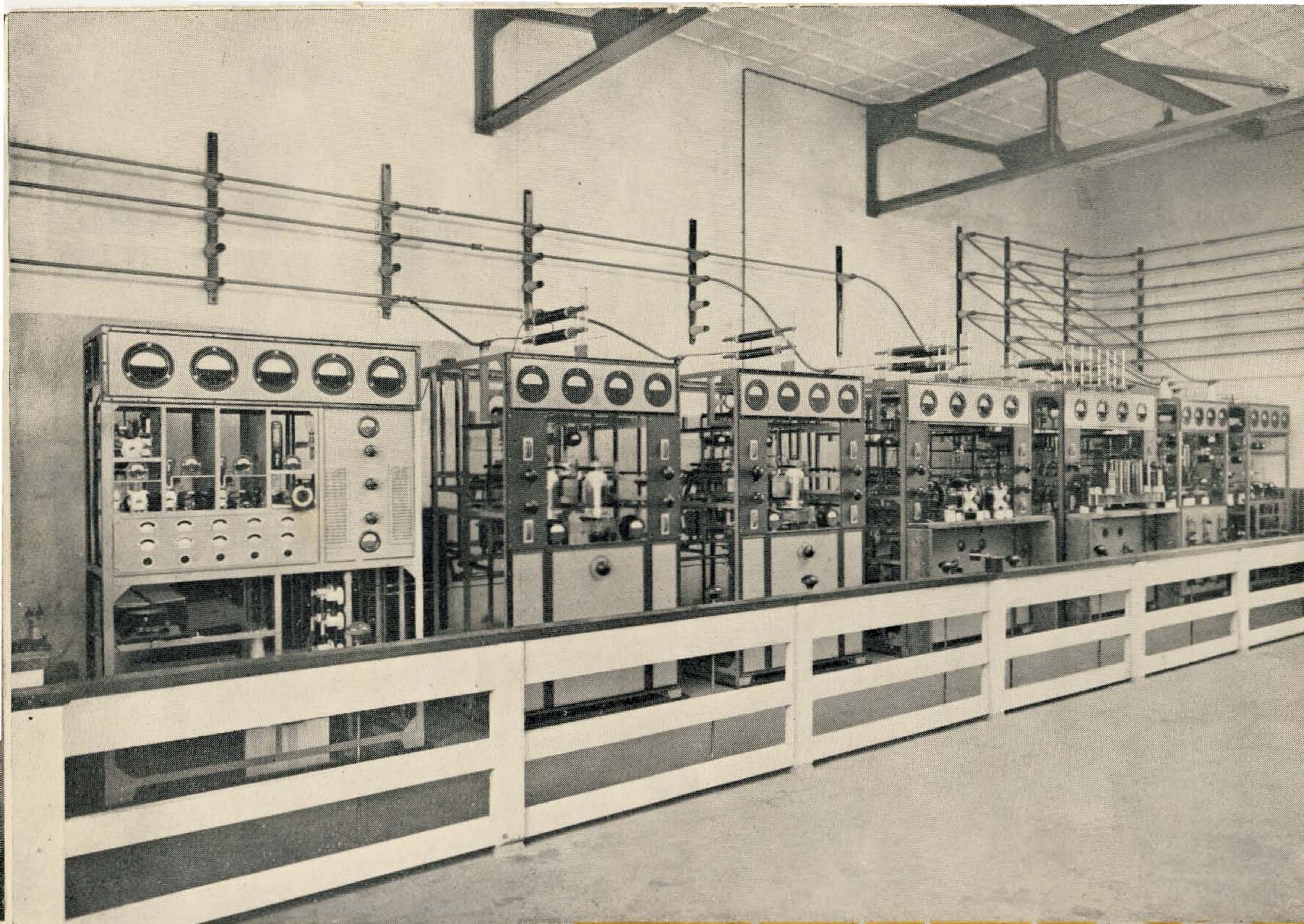
Totaal-overzicht van den zender.
