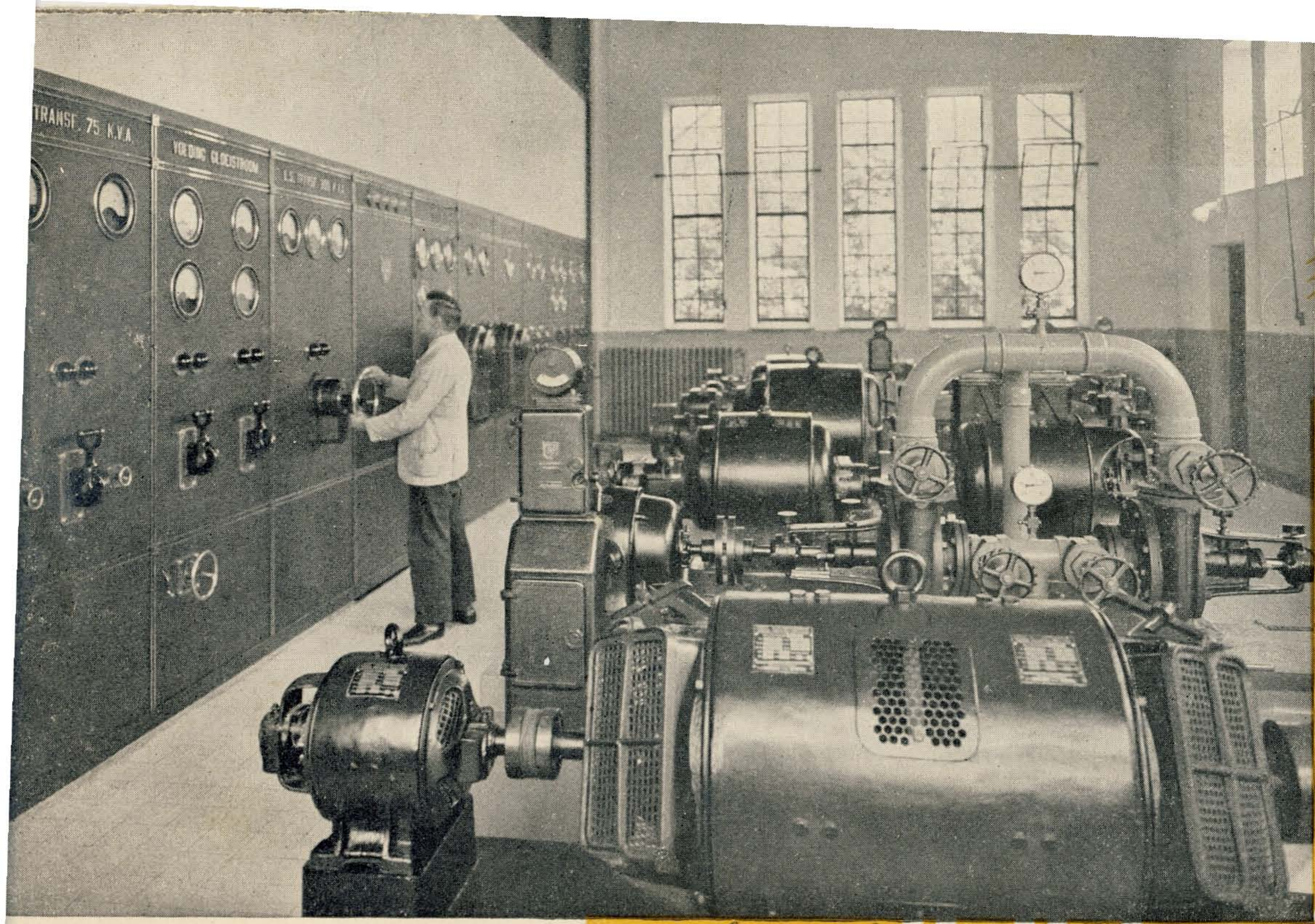
De machinekamer met koelwaterpompen.
