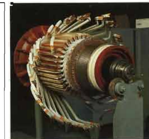
tractiemotoren (locatie Electrorail NV - Utrecht)
