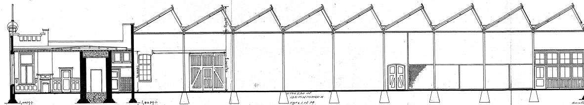
DOORSNED E. A. B.
